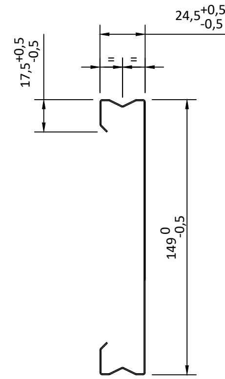
SEZIONE A-A
