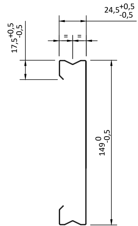
SEZIONE A-A
