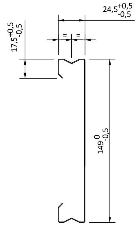
SEZIONE A-A
